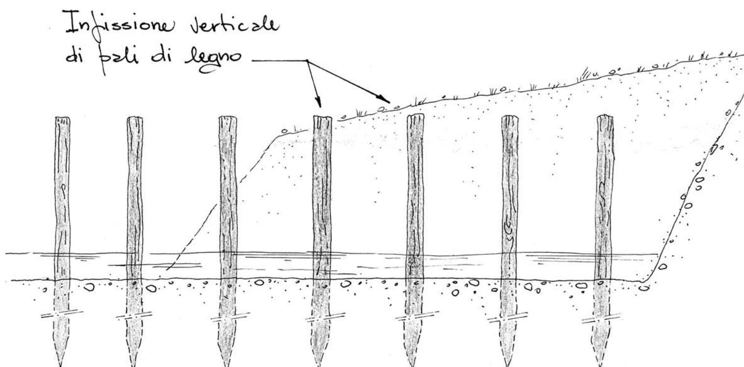
Dis. 4 - Repellente vivo di ramaglia a strati. Fase 3 (sezione).
