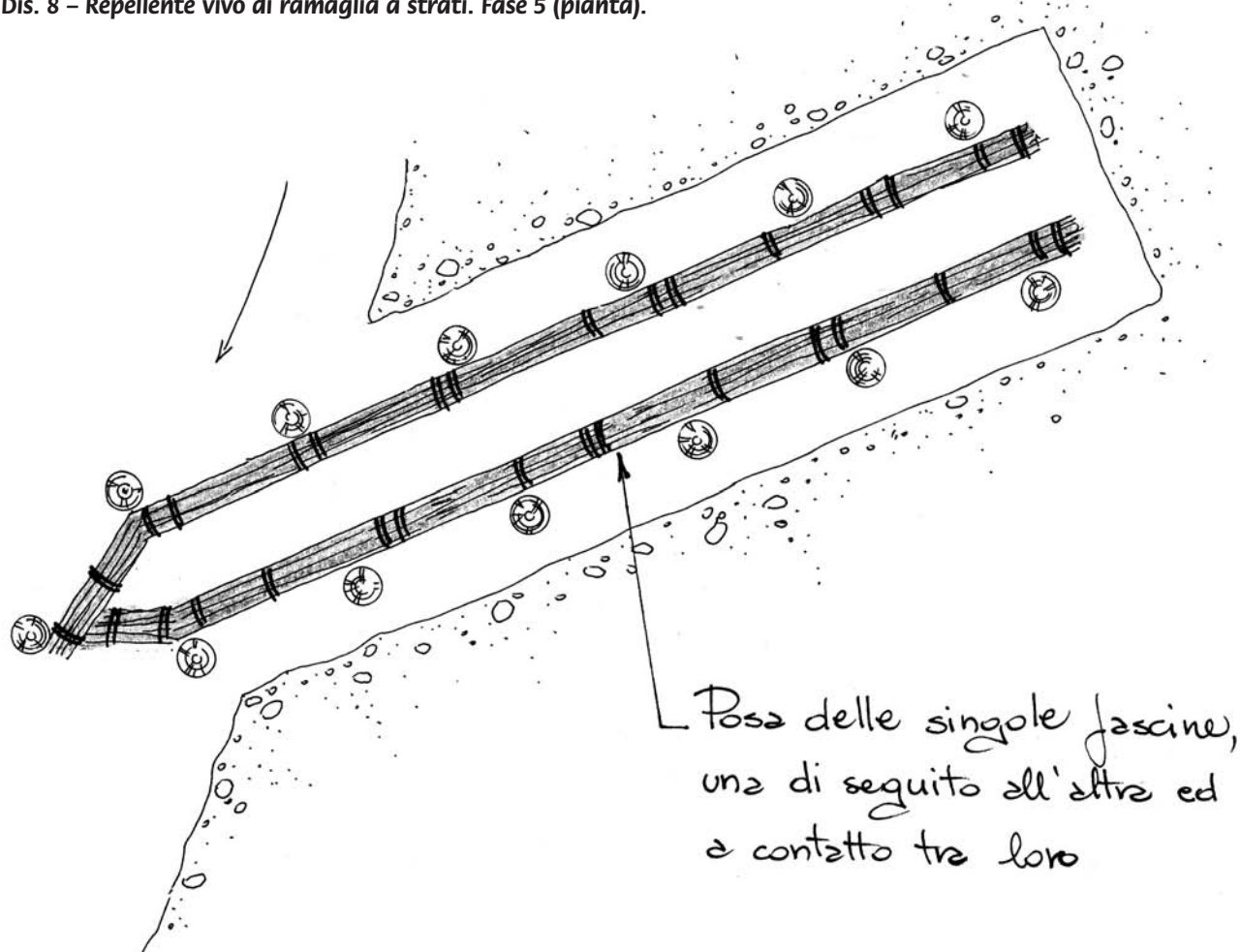
Dis. 8 – Repellente vivo di ramaglia a strati. Fase 5 (pianta).
