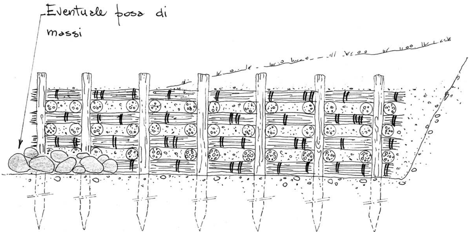
Dis. 17 – Repellente vivo di ramaglia a strati. Fase 10 (sezione).
