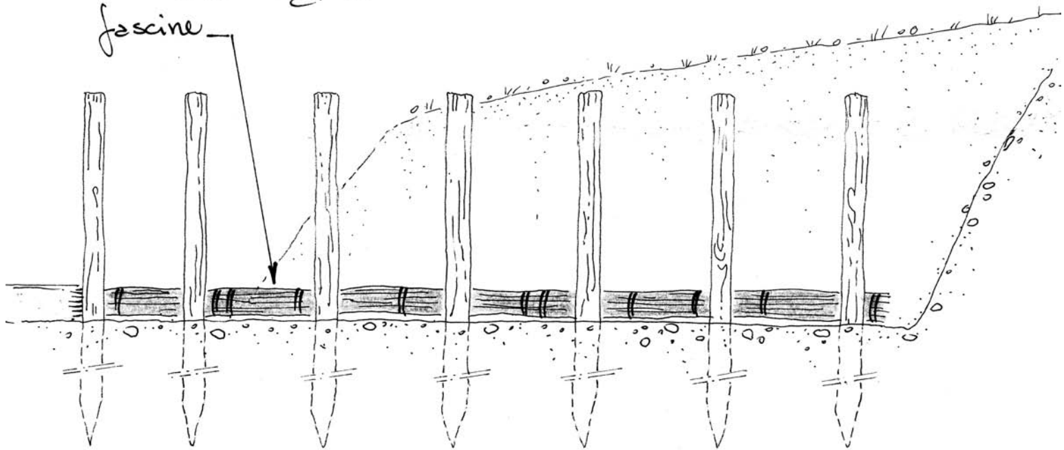
Dis. 7 – Repellente vivo di ramaglia a strati. Fase 5 (sezione).
