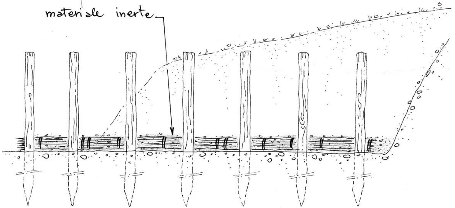
Dis. 9 - Repellente vivo di ramaglia a strati. Fase 6 (sezione).
