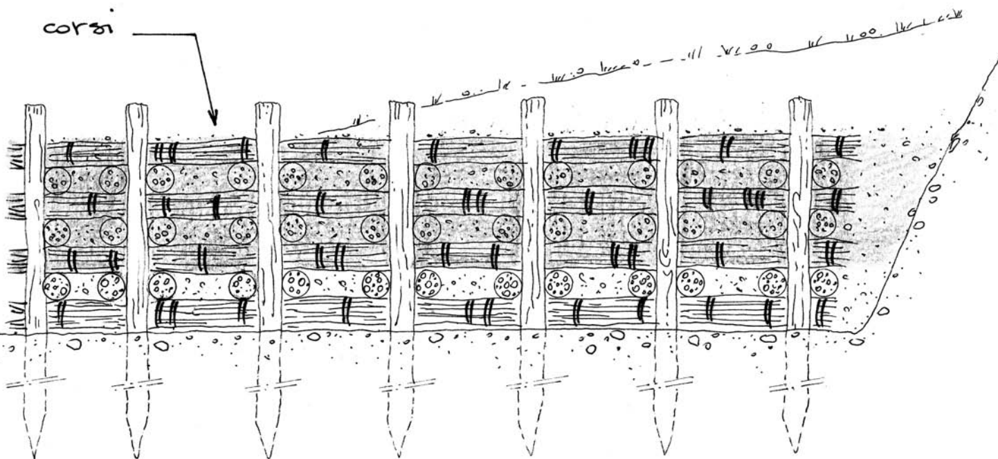
Dis. 15 - Repellente vivo di ramaglia a strati. Fase 9 (sezione).
