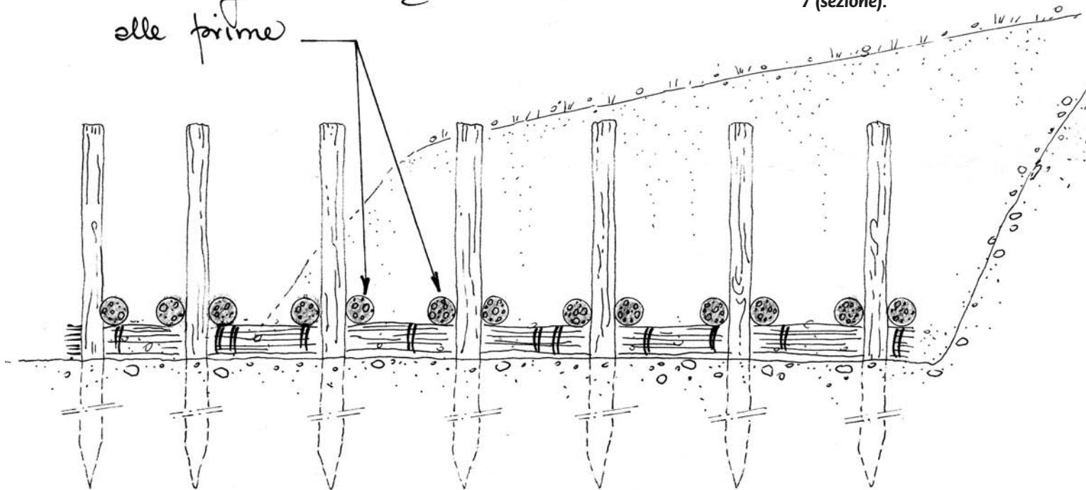
Dis. 11 - Repellente vivo di ramaglia a strati. Fase 7 (sezione).
