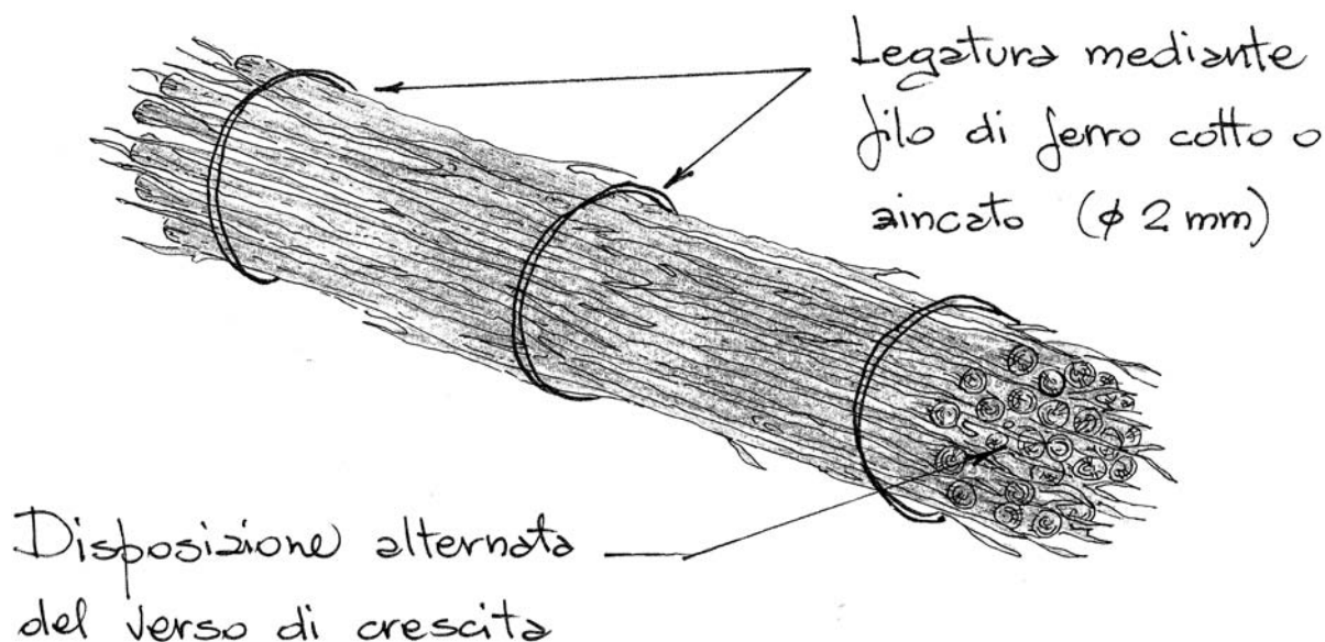
Dis. 6 – Repellente vivo di ramaglia a strati. Fase 4 (particolare).
