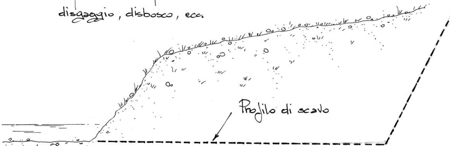
Dis. 1 - Repellente vivo di ramaglia a strati. Fase 1 - Ipotetica situazione di dissesto con evidenziati gli elementi morfologici più caratteristici e le operazioni da eseguirsi (in tratteggio il profilo di scavo) (sezione).
