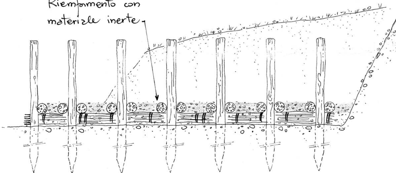
Dis. 13 – Repellente vivo di ramaglia a strati. Fase 8 (sezione).
