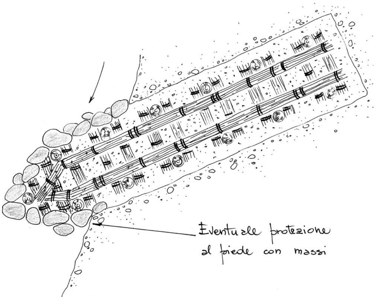
Dis. 18 – Repellente vivo di ramaglia a strati. Fase 10 (pianta).
