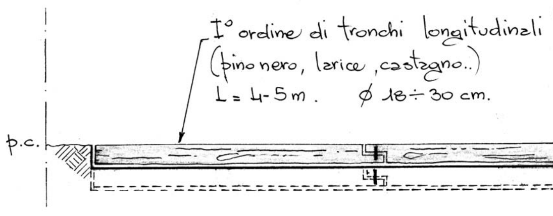
Dis. 7 - Palificata viva doppia (di versante). Fase 3 (vista frontale).
