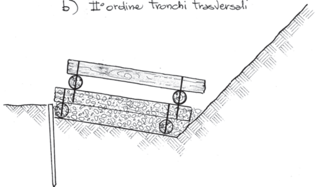
Dis. 19 - Palificata viva doppia (di versante). Fase 6 (sezione).
