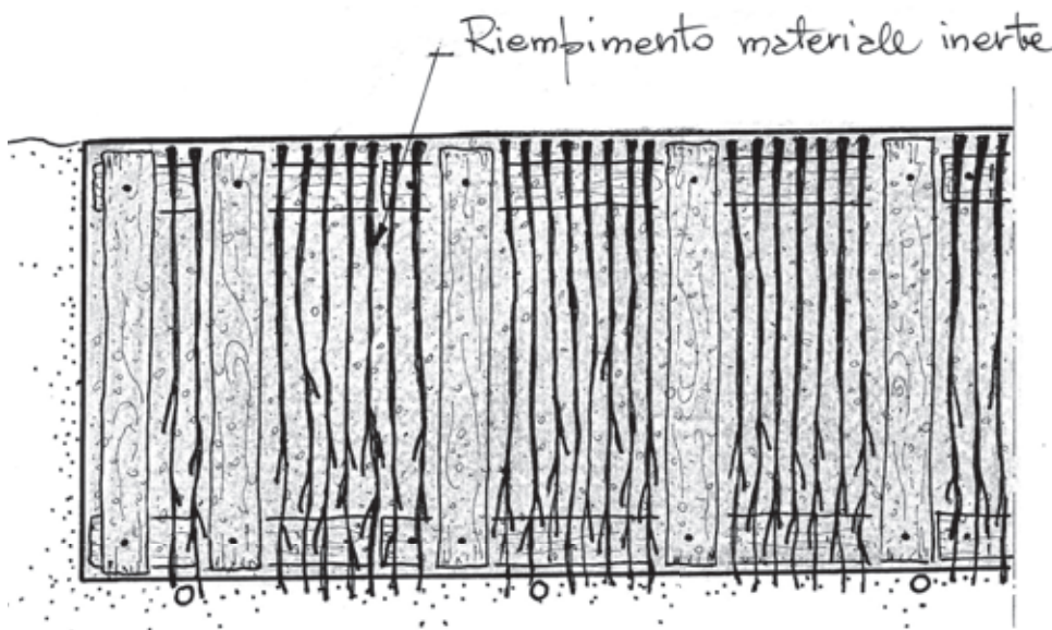
Dis. 33 - Palificata viva doppia (di versante). Fase 9 (pianta).
