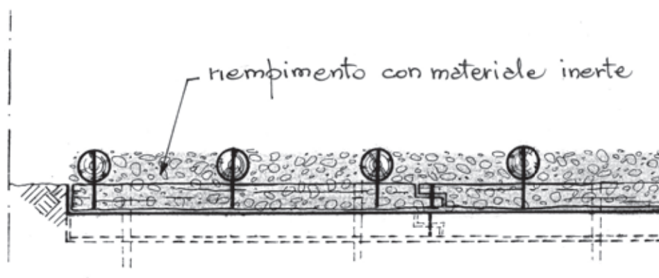
Dis. 17 – Palificata viva doppia (di versante). Fase 5 (vista frontale).
