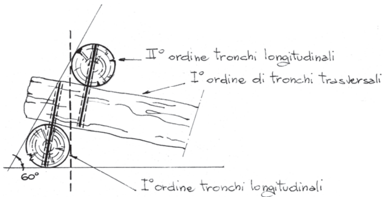
Dis. 22 – Palificata viva doppia (di versante). Fase 6 - Arretramento delle file di tronchi longitudinali (correnti) rispetto alle sottostanti (particolare; sezione).
