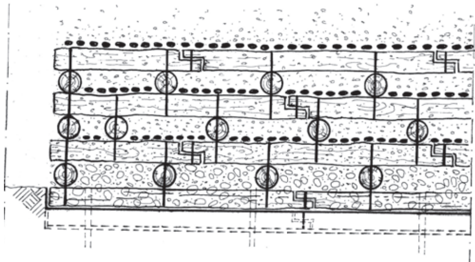
Dis. 36 – Palificata viva doppia (di versante). Fase 10 (vista frontale).
