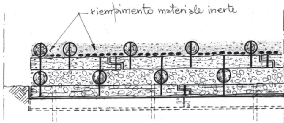
Dis. 32 - Palificata viva doppia (di versante). Fase 9 (vista frontale).
