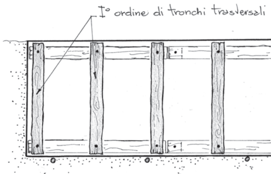
Dis. 12 – Palificata viva doppia (di versante). Fase 4 (pianta).
