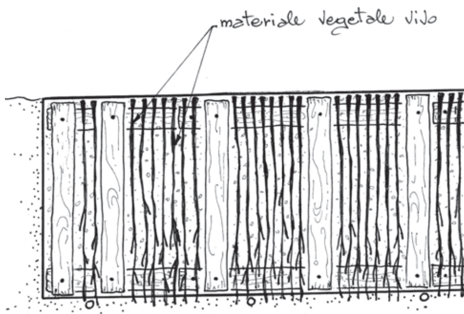
Dis. 29 - Palificata viva doppia (di versante). Fase 8 (pianta).
