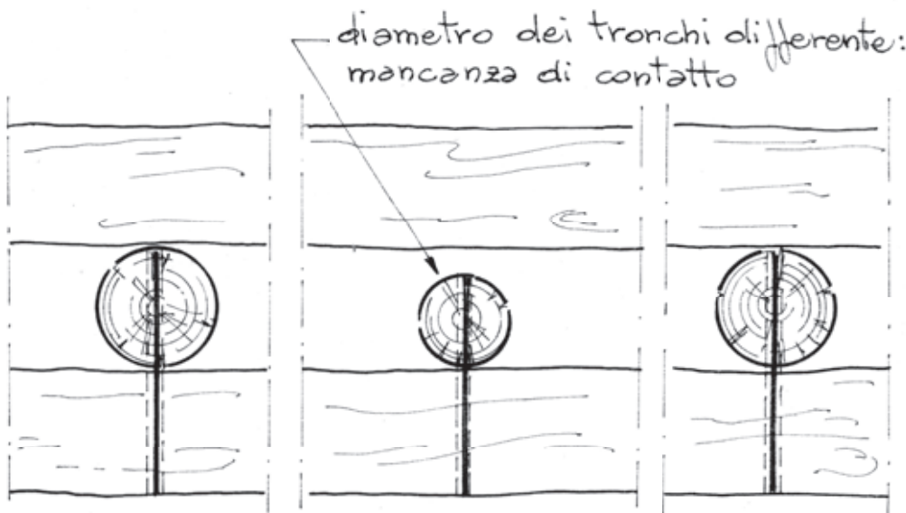
Dis. 13 - Palificata viva doppia (di versante). Fase 4 - Scelta degli elementi trasversali: i diametri devono essere compatibilmente simili (particolare; vista frontale).
