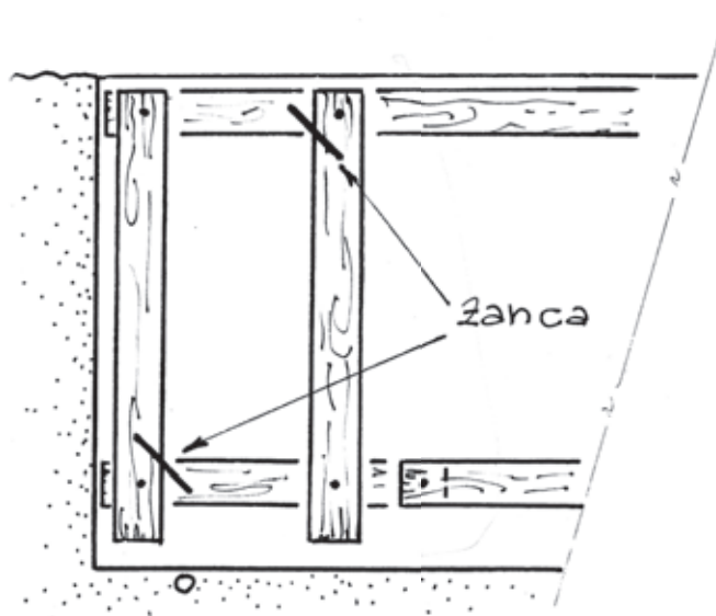
Dis. 15 – Palificata viva doppia (di versante). Fase 4 - Fissaggio provvisorio (particolare; sezione, pianta).
