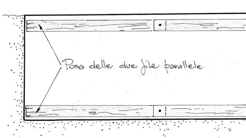
Dis. 8 – Palificata viva doppia (di versante). Fase 3 (pianta).
