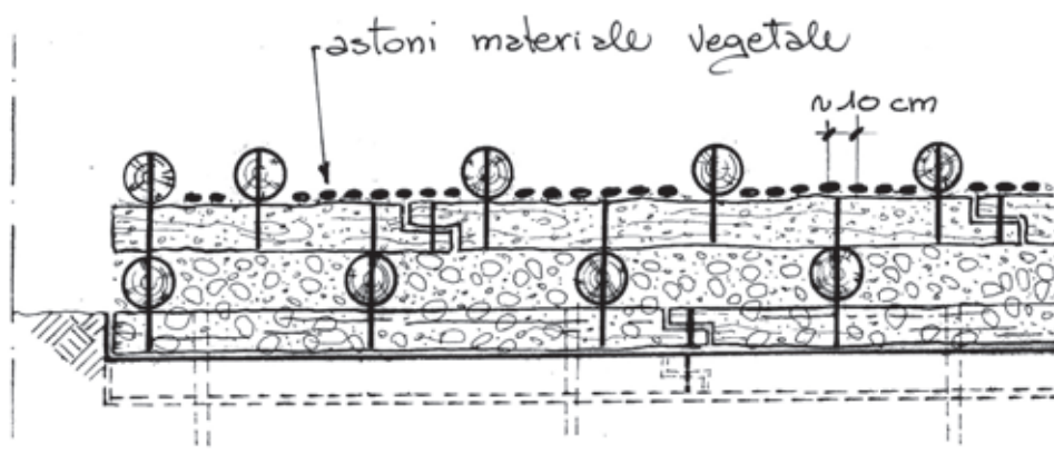
Dis. 28 - Palificata viva doppia (di versante). Fase 8 (vista frontale).
