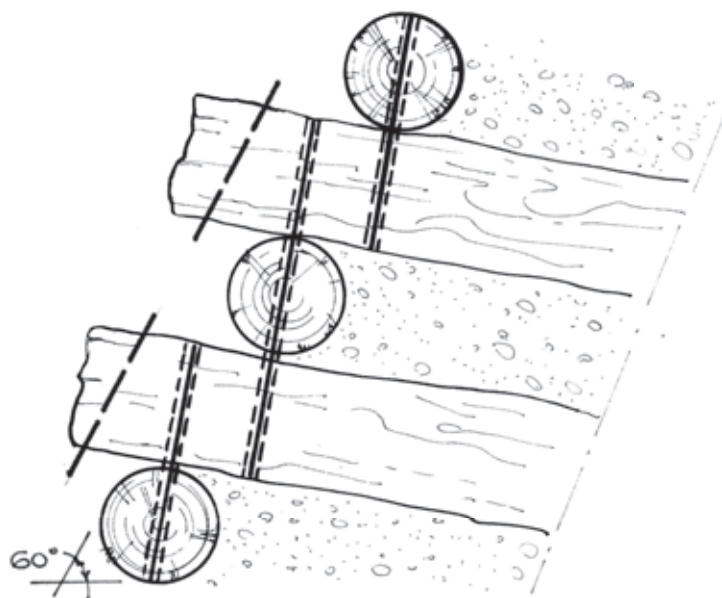
Dis. 38 – Palificata viva doppia (di versante). Fase 11 - Sagomatura dei tronchi trasversali troppo sporgenti (particolare; sezione).
