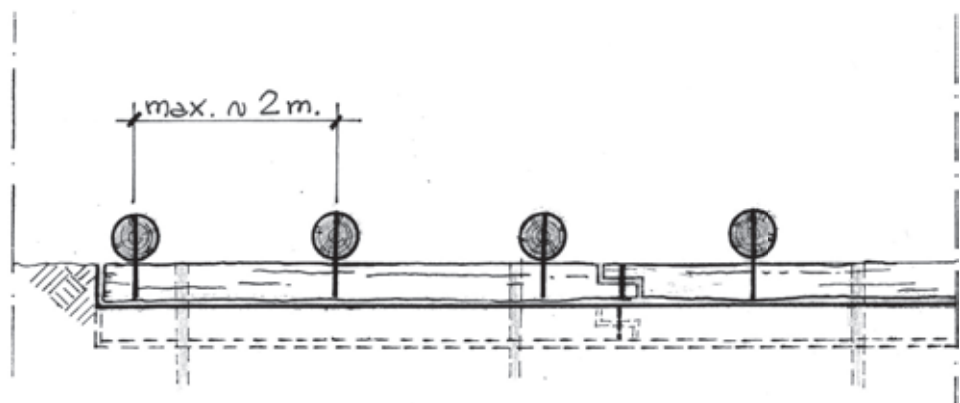
Dis. 11 - Palificata viva doppia (di versante). Fase 4 (vista frontale).
