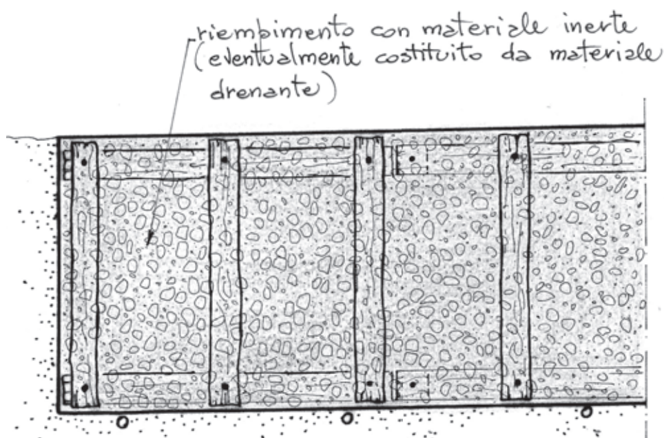
Dis. 18 – Palificata viva doppia (di versante). Fase 5 (pianta).
