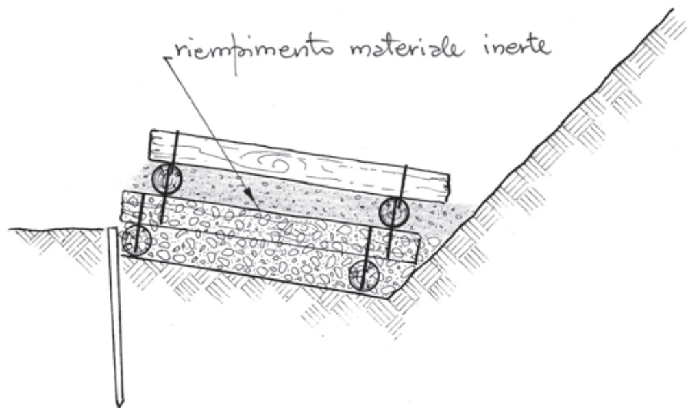
Dis. 25 – Palificata viva doppia (di versante). Fase 7 (vista frontale).
