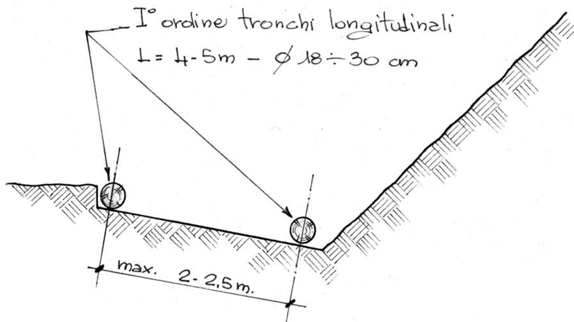
Dis. 6 - Palificata viva doppia (di versante). Fase 3 (sezione).
