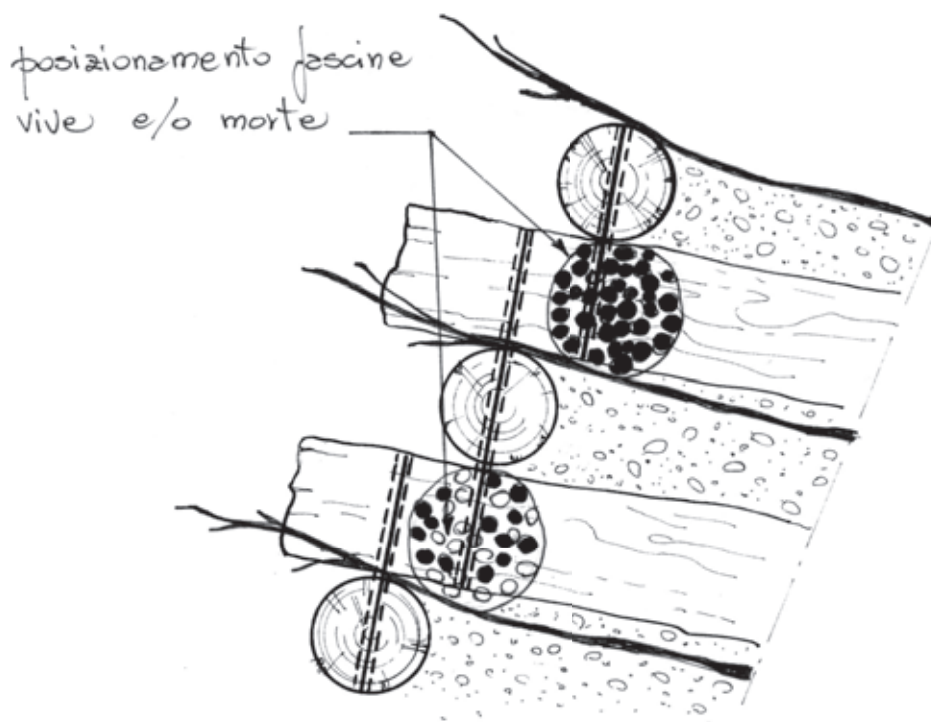
Dis. 34 – Palificata viva doppia (di versante). Fase 9 - Posizionamento di fascine (vive o morte o miste) dietro la parete esterna a contenimento del materiale di riempimento (particolare; sezione).
