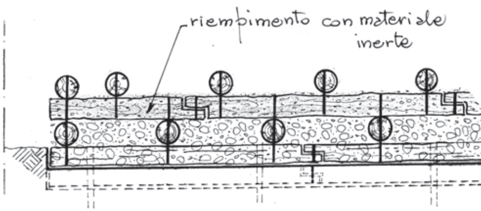
Dis. 25 – Palificata viva doppia (di versante). Fase 7 (vista frontale).
