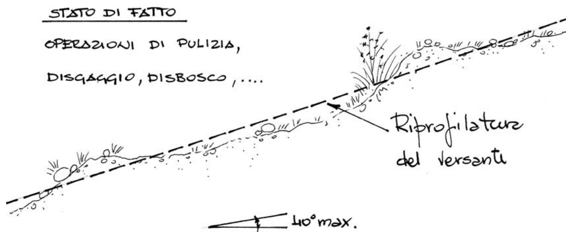
Dis. 1 – Gradonata viva. Fase 1 - Ipotetica situazione di dissesto con evidenziati gli elementi morfologici più caratteristici e le operazioni da eseguirsi (in tratteggio la riprofilatura ed il rimodellamento del versante) (sezione).
