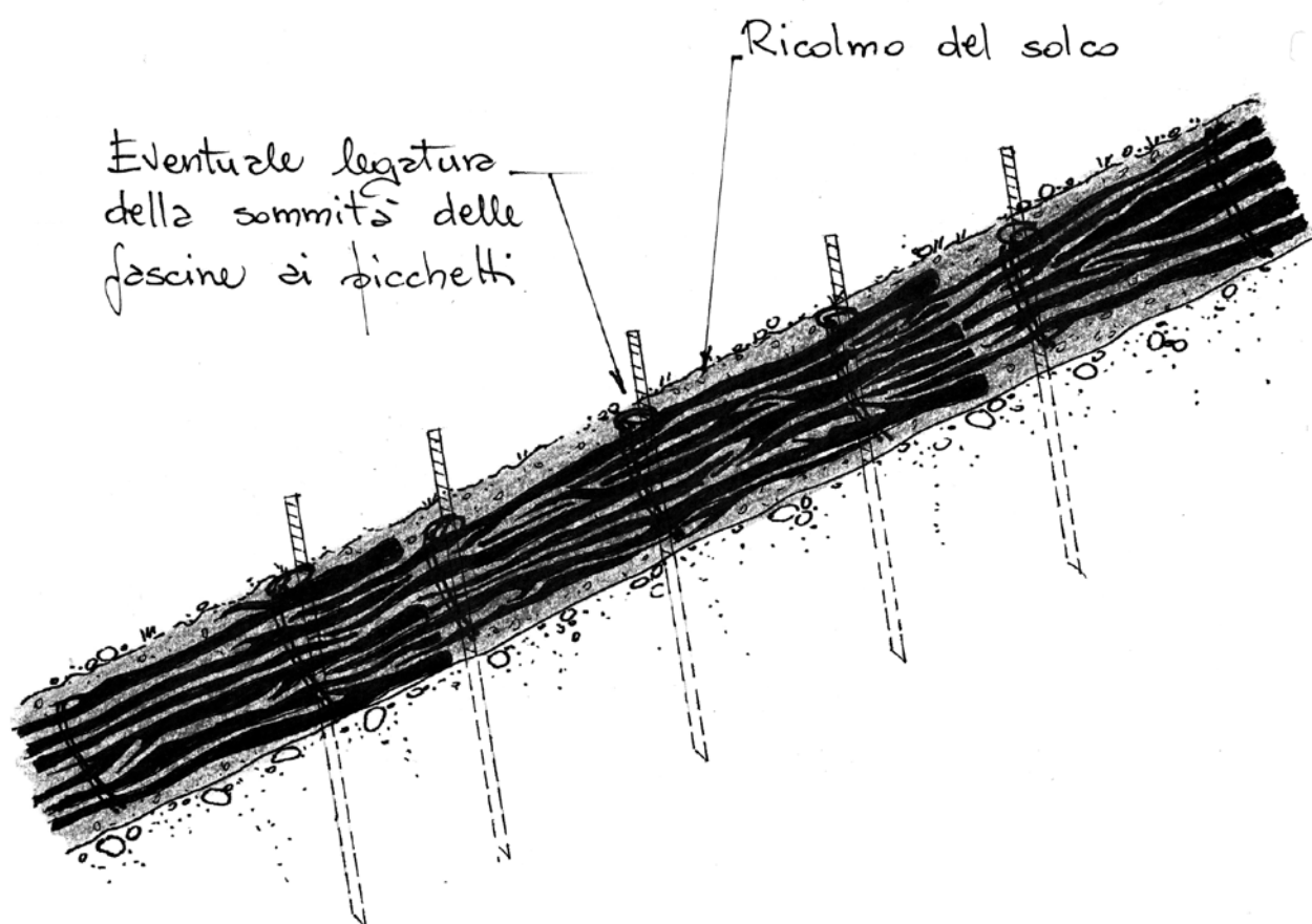
Dis. 6 - Fascinata viva drenante. Fase 6 (sezione).
