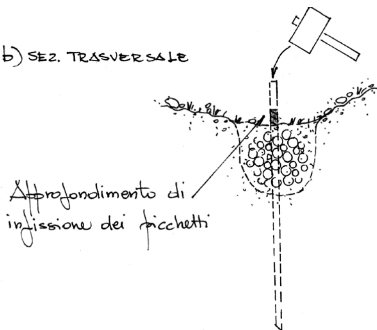
Dis. 7 - Fascinata viva drenante. Fase 7 (sezione).
