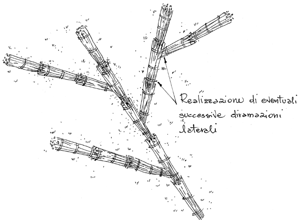
Dis. 8 – Fascinata viva drenante. Fase 8 (schema).
