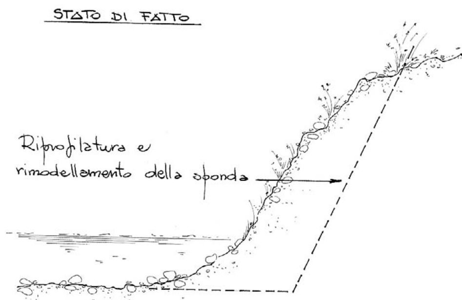
Dis. 1 - Gabbionata in rete metallica zincata rinverdata (di versante e spondale). Fase 1 - Ambito fluviale. Ipotetica situazione di dissesto con evidenziati gli elementi morfologici più caratteristici e le operazioni da eseguirsi (in tratteggio la riprofilatura ed il rimodellamento della sponda) (sezione).
