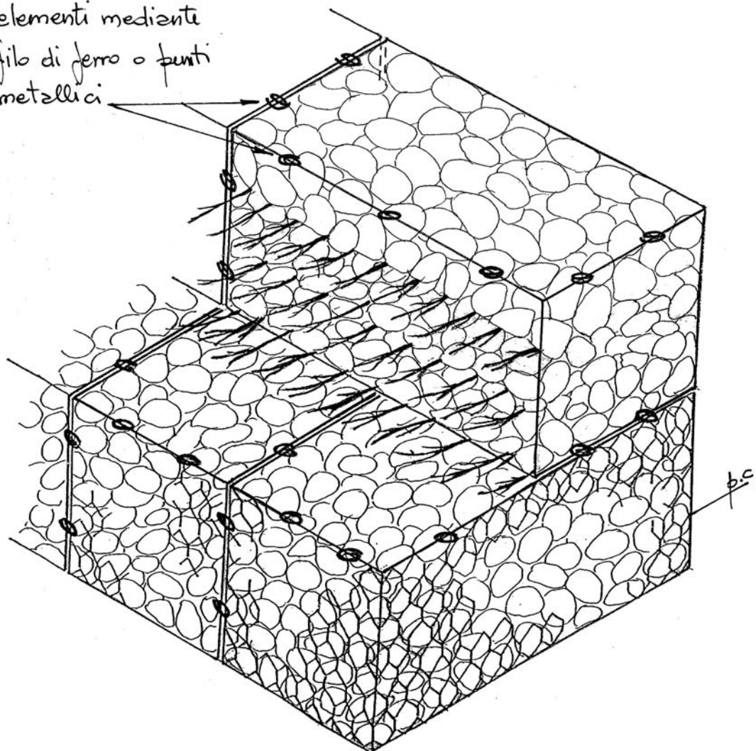
Dis. 15 – Gabbionata in rete metallica zincata rinverdita (di versante e spondale). Fase 9 - Ambito terrestre (assonometria).
