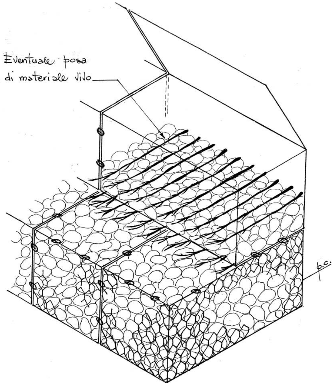
Dis. 12 – Gabbionata in rete metallica zincata rinverdita (di versante e spondale). Fase 8 - Ambito terrestre (assonometria).
