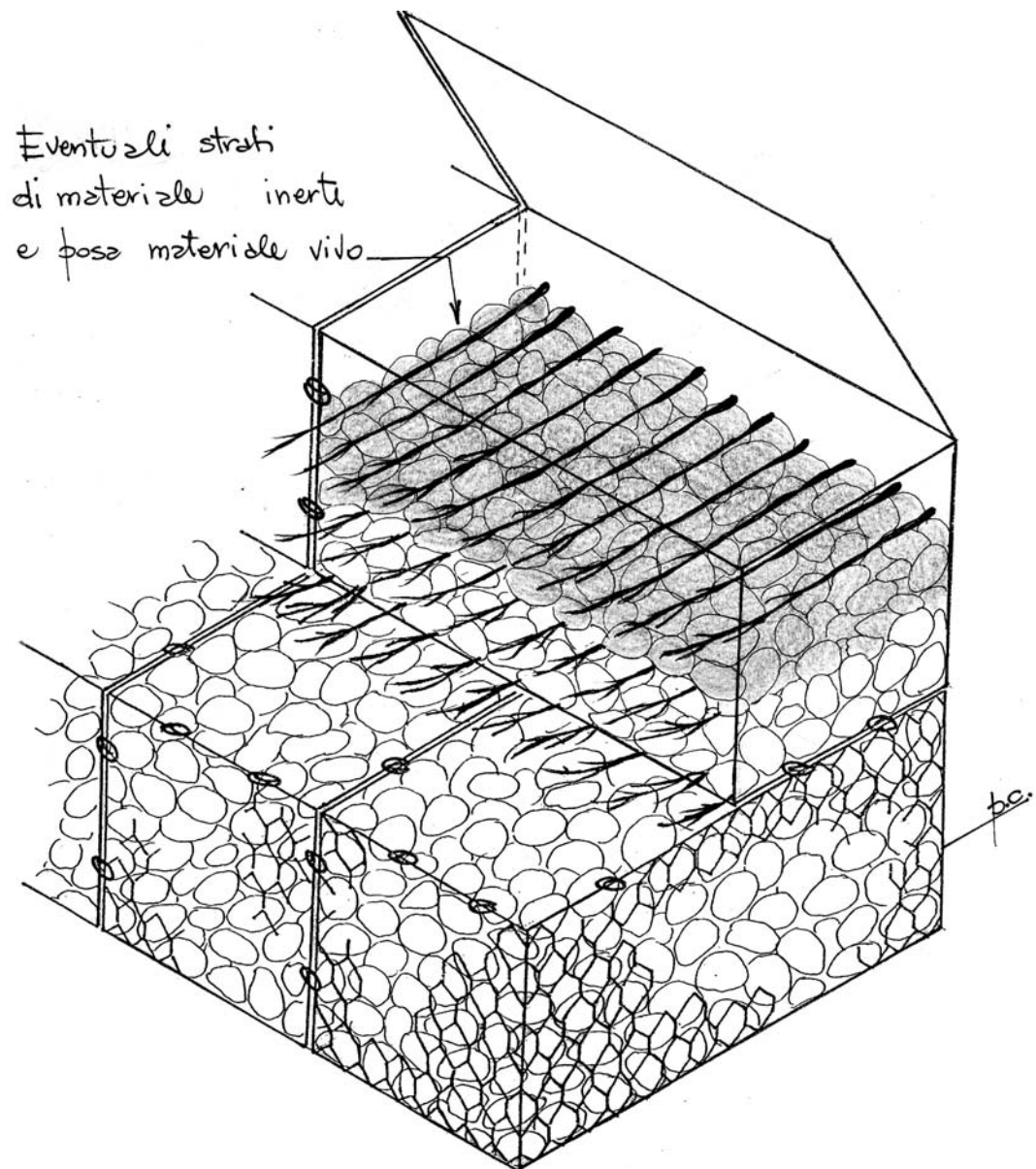
Dis. 13 – Gabbionata in rete metallica zincata rinverdita (di versante e spondale). Fase 8 - Ambito terrestre (assonometria).
