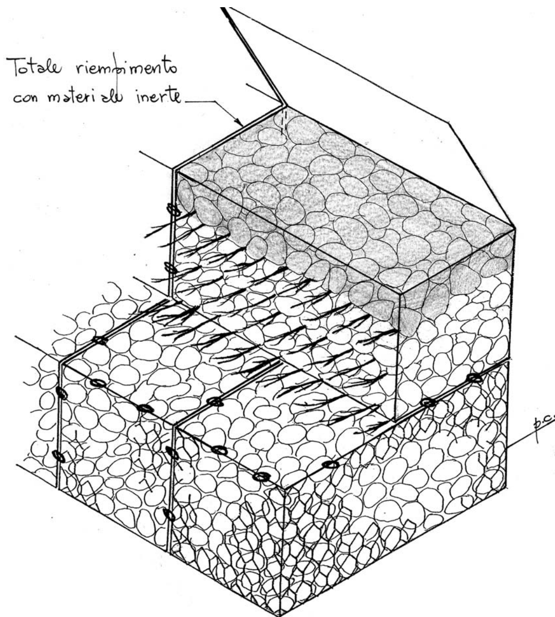
Dis. 14 – Gabbionata in rete metallica zincata rinverditata (di versante e spondale). Fase 8 - Ambito terrestre (assonometria).
