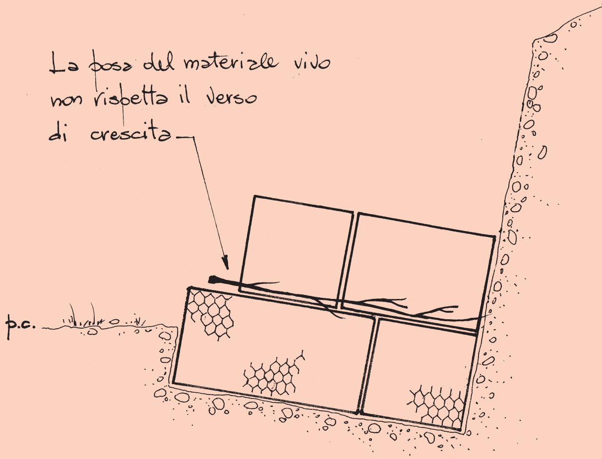
Dis. 10 – Gabbionata in rete metallica zincata rinverdata (di versante e spondale). Fase 7 - Ambito terrestre. Posa non rispettosa del verso di crescita del materiale vegetale vivo negli elementi ("gabbioni") (sezione).
