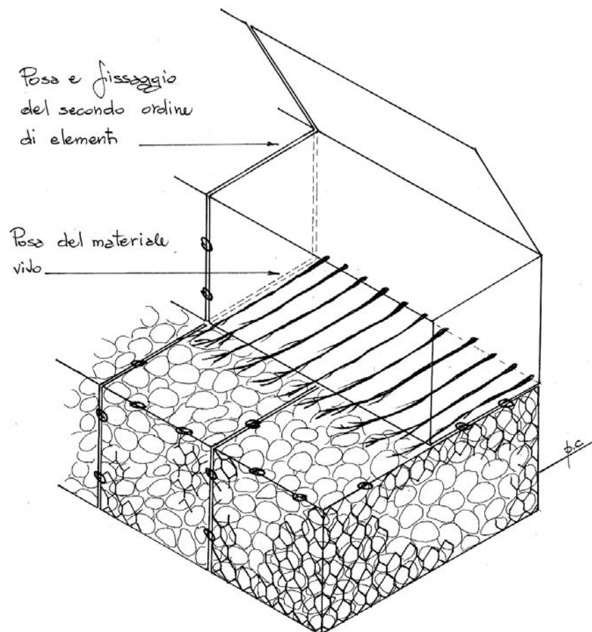
Dis. 9 - Gabbionata in rete metallica zincata rinverditata (di versante e spondale). Fase 7 - Ambito terrestre (assonometria).
