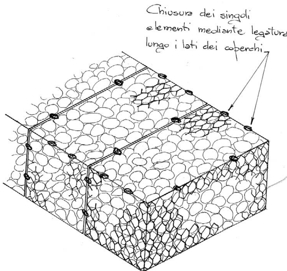
Dis. 8 - Gabbionata in rete metallica zincata rinverdata (di versante e spondale). Fase 5 - Ambito terrestre (assonometria).
