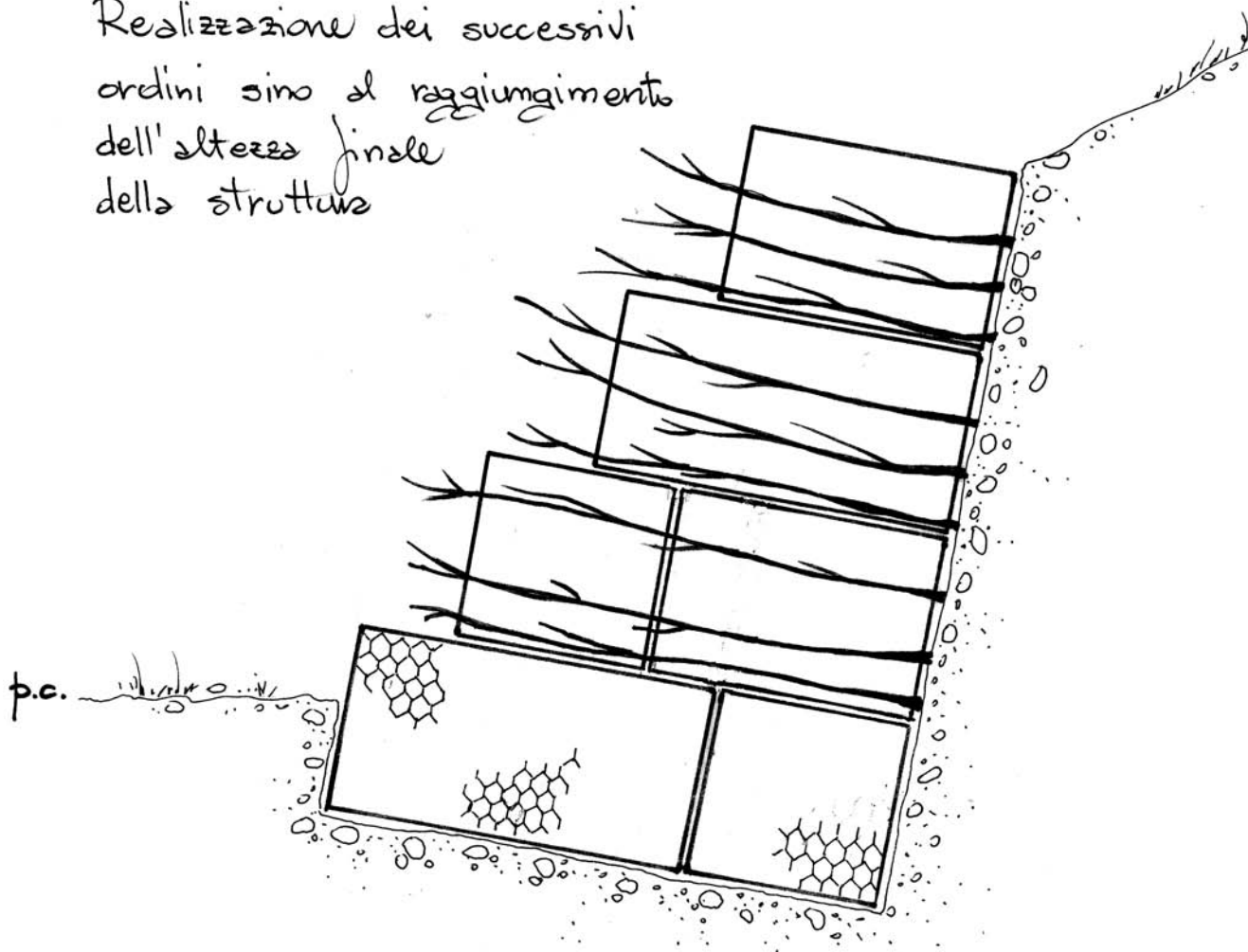
Dis. 16 – Gabbionata in rete metallica zincata rinverdita (di versante e spondale). Fase 10 - Ambito terrestre (sezione).
