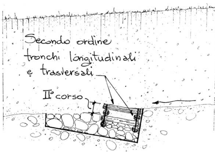
Dis. 21 – Briglia viva in legname e pietrame. Fase 7 (sezione).
