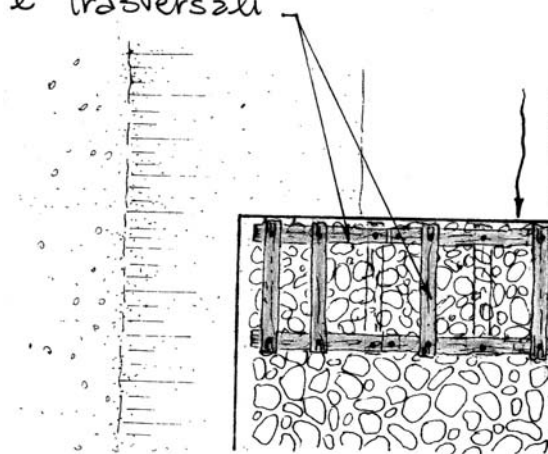
Dis. 23 – Briglia viva in legname e pietrame. Fase 7 (pianta).
