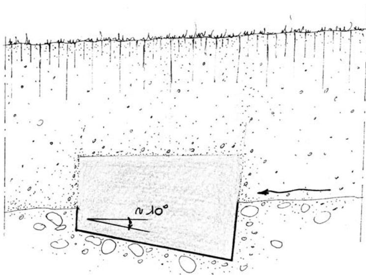
Dis. 2 - Briglia viva in legname e pietra- me. Fase 2 (sezione).
