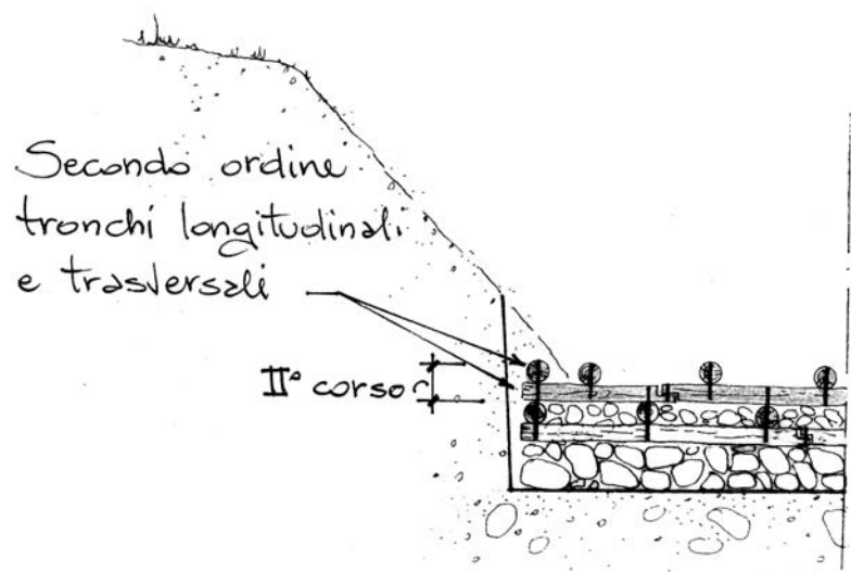
Dis. 22 – Briglia viva in legname e pietrame. Fase 7 (vista frontale).
