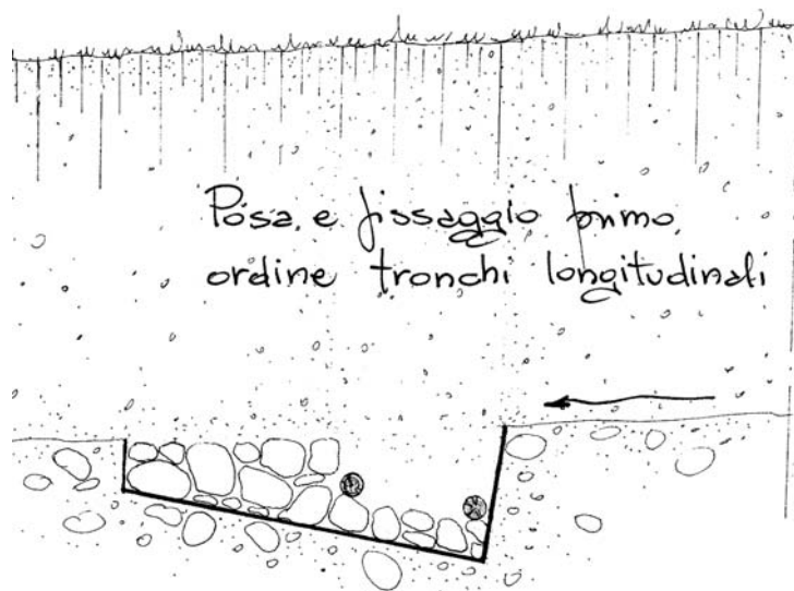
Dis. 8 – Briglia viva in legname e pietrame. Fase 4 (sezione).
