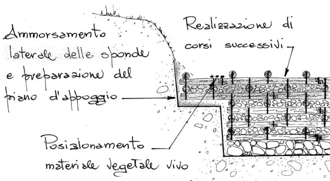
Dis. 32 - Briglia viva in legname e pietrame. Fase 10 (vista frontale).
