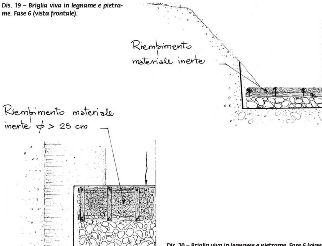
Dis. 20 – Briglia viva in legname e pietrame. Fase 6 (pianta).
