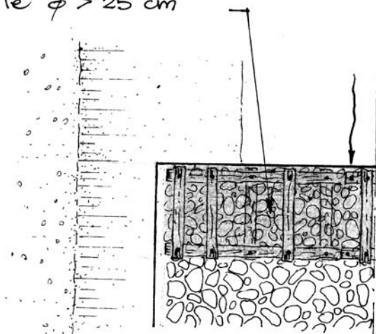
Dis. 27 – Briglia viva in legname e pietrame. Fase 8 (pianta).
