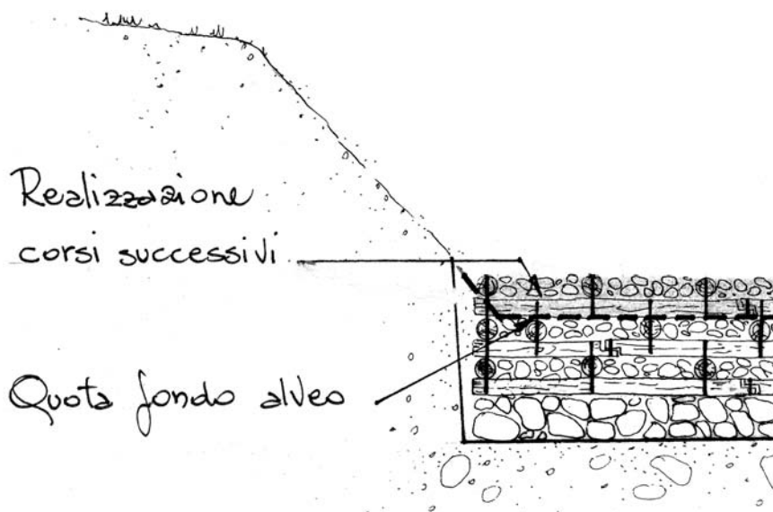
Dis. 29 - Briglia viva in legname e pietrame. Fase 9 (vista frontale).
