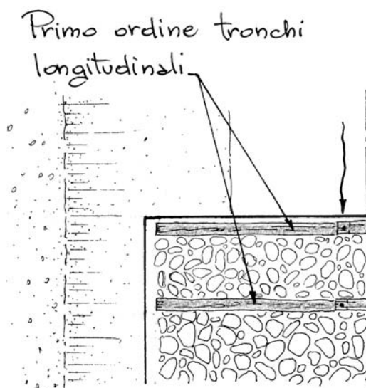
Dis. 10 – Briglia viva in legname e pietrame. Fase 4 (pianta).
