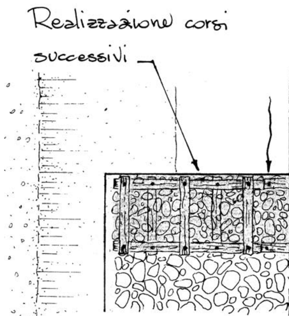
Dis. 30 - Briglia viva in legname e pietrame. Fase 9 (pianta).
