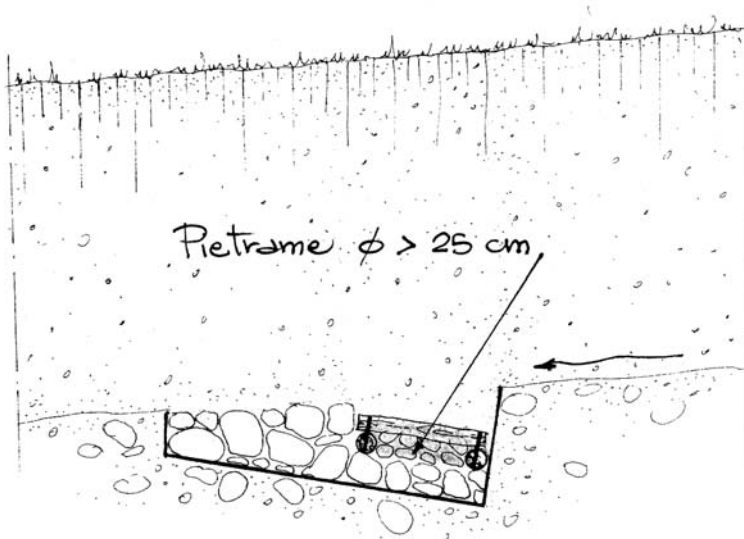
Dis. 18 – Briglia viva in legname e pietrame. Fase 6 (sezione).
