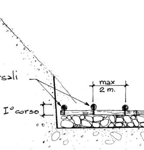
Dis. 13 – Briglia viva in legname e pietrame. Fase 5 (vista frontale).
