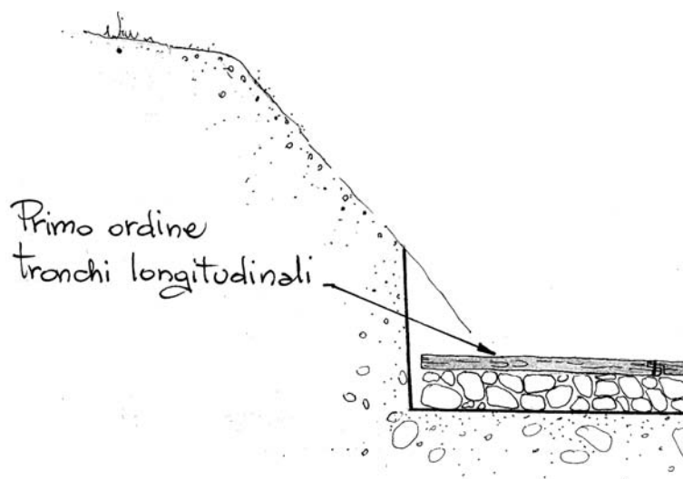
Dis. 9 – Briglia viva in legname e pietrame. Fase 4 (vista frontale).
