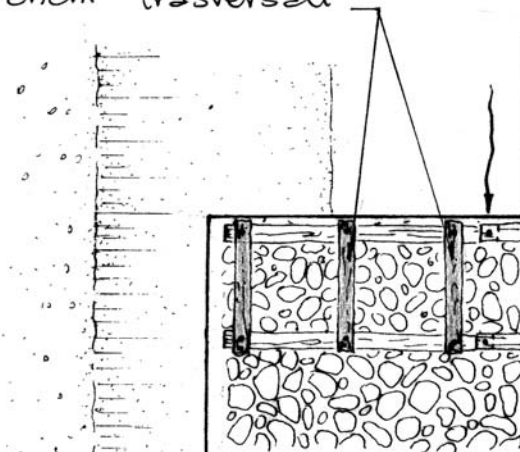
Dis. 14 – Briglia viva in legname e pietrame. Fase 5 (pianta).
