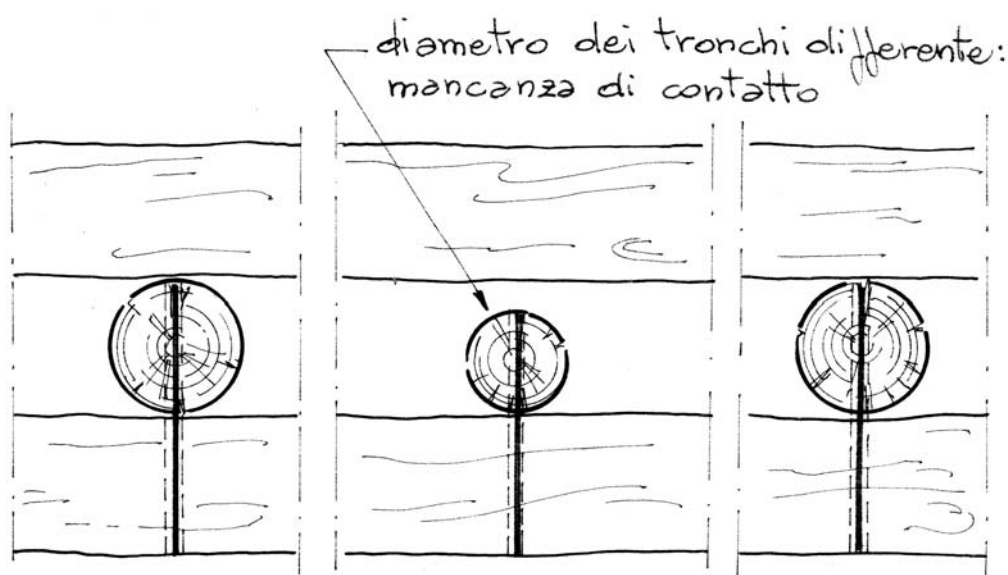
Dis. 15 - Briglia viva in legname e pietrame. Fase 5 - Scelta degli elementi trasversali: i diametri devono essere compatibilmente simili (particolare; vista frontale).
