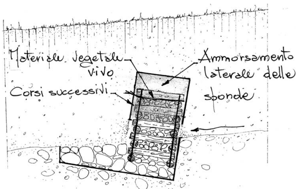
Dis. 31 - Briglia viva in legname e pietrame. Fase 10 (sezione).
