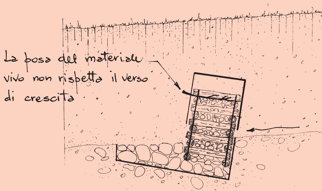
Dis. 34 – Briglia viva in legname e pietrame. Fase 10 - Posa non rispettosa del verso di crescita del materiale vegetale vivo (sezione).
