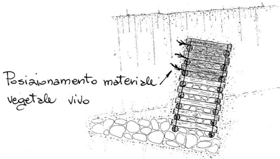
Dis. 35 - Briglia viva in legname e pietrame. Fase 11 (sezione).
