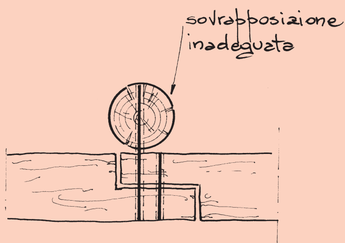
Dis. 24 – Briglia viva in legname e pietrame. Fase 7 - Sovrapposizioni di incastri e chiodature (particolare; vista frontale).
