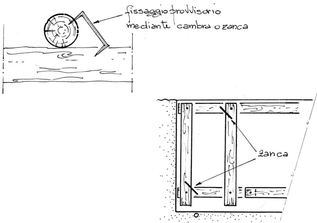
Dis. 17 – Briglia viva in legname e pietrame. Fase 5 - Fissaggio provvisorio (particolare; sezione, pianta).
