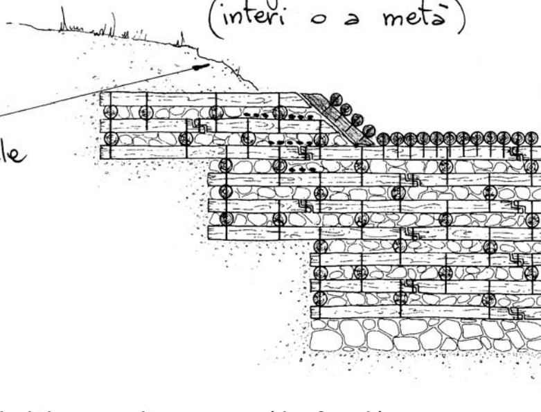
Dis. 36 – Briglia viva in legname e pietrame. Fase 11 (vista frontale).
