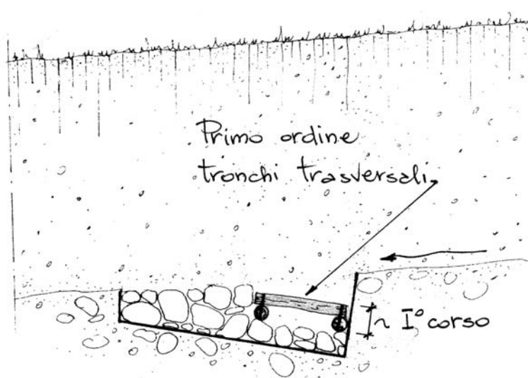
Dis. 12 – Briglia viva in legname e pietra. Fase 5 (sezione).
